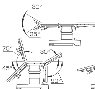
Механический встроенный почечный валик (опция)
