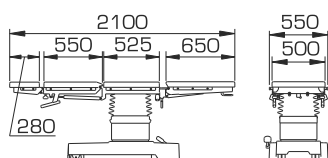
Механический излом спинной секции (опция)
